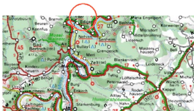
Mosel Verlauf - ab Ediger-Eller
